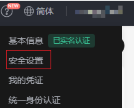
图 8-31 安全设置
