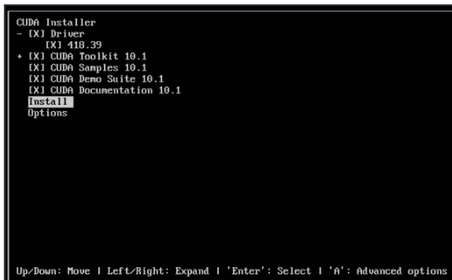
图 2-133 安装 CUDA_2
