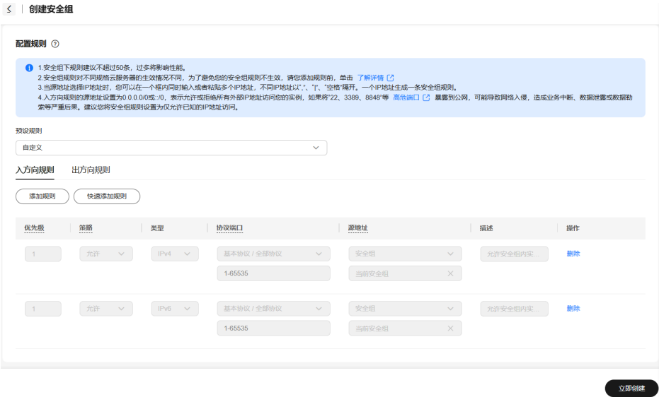
图 8-13 配置规则
