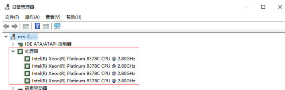
图 2-157 查询结果
