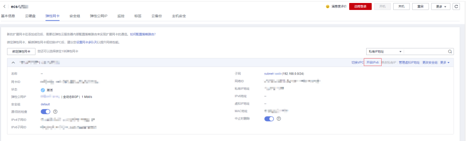
图 6-7 开启 IPv6
