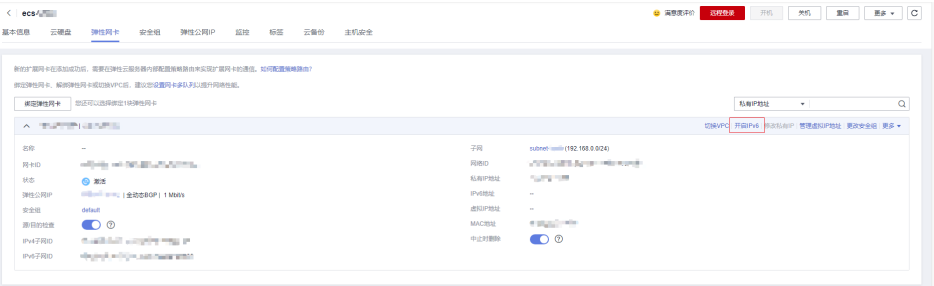
图 6-9 开启 IPv6
