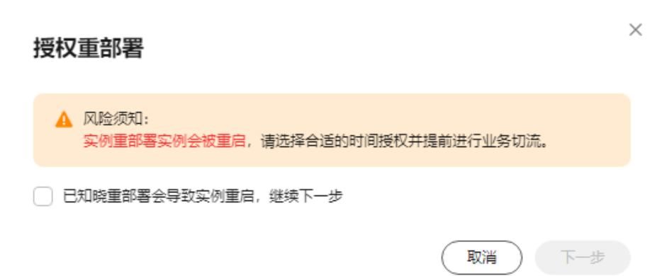
图 13-3 授权重部署
