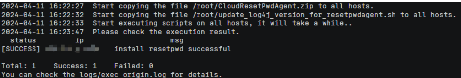
图 10-29 运行成功
