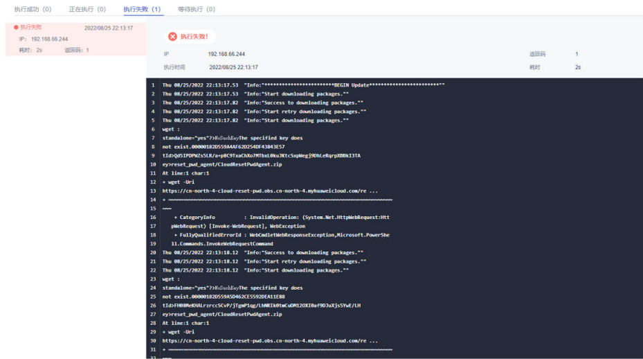
图 10-26 执行失败
