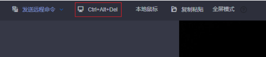
图 2-28 单击“Ctrl+Alt+Del”
