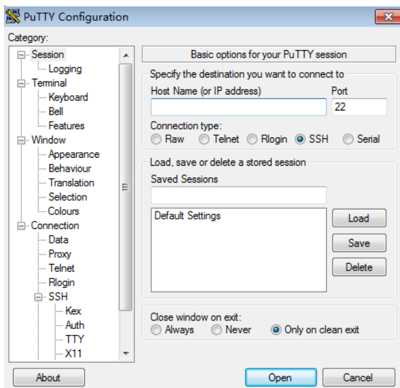
图 2-71 单击“Session”
