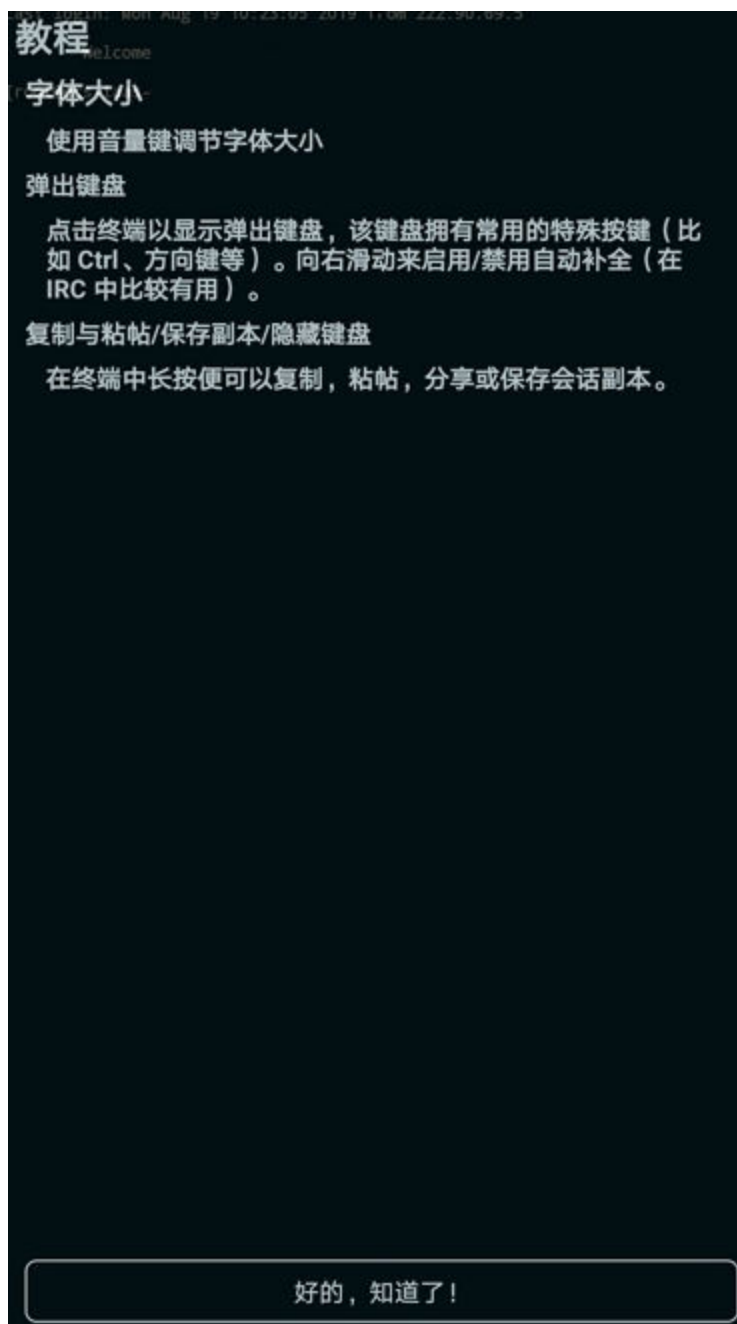
图 2-82 教程
