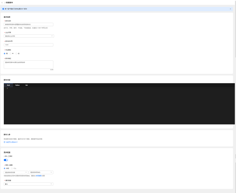
图 10-22 创建脚本
