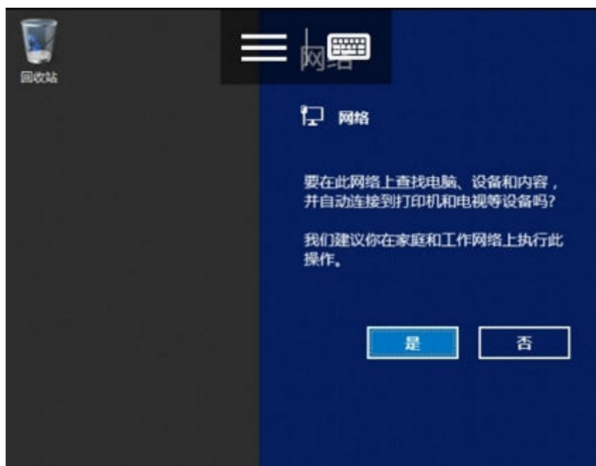
图 2-45 登录成功
